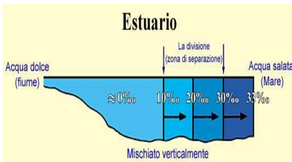
Figura 14: Sezione longitudinale che mostra la salinità (in millesimi di percentuale) in un estuario. È possibile vedere qui la divisione (zona di separazione) tra l'acqua dolce e quella salata. ( Introductory Oceanography (Introduzione all'Oceanografia), Thurman, p. 301, (con un piccolo miglioramento.)
