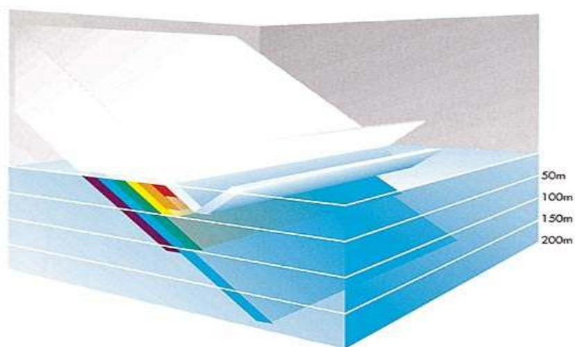
Figura 15: Una percentuale che varia dal 3 al 30% della luce solare viene riflessa dalla superficie del mare. Al di sotto della superficie quasi tutti i 7 colori dello spettro sono assorbiti uno dopo l'altro nei primi 200 metri, tranne il blu. ( Oceans (Oceani), Elder e Pernetta, p. 27.)
