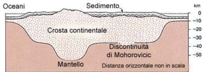
Figura 7: Le montagne possiedono radici profonde sotto la superficie della terra. ( Earth (Terra), Press e Siever, p. 413.)
