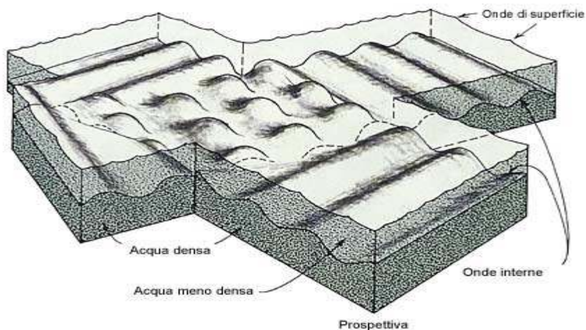
Figura 16: Onde interne sull'interfaccia che si trova tra due strati d'acqua di diversa densità. Una è densa (la più profonda), l'altra è meno densa (la più superficiale). ( Oceanography (Oceanografia), Gross, p. 204.)
