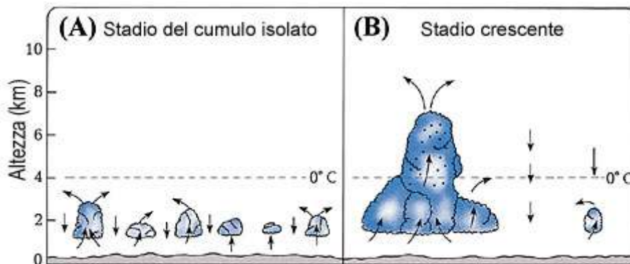
Figura 19: (A) Piccole nubi isolate (nubi cumulo). (B) Quando le piccole nubi si uniscono, le correnti ascensionali all'interno della grossa nube aumentano, così la nuvola si ingrandisce. Le gocce di pioggia sono indicate con •. ( The Atmosphere (Atmosfera), Anthes ed altri, p. 269.)
