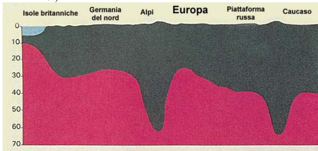
Figura 8: Sezione schematica. Le montagne, come pioli, penetrano profondamente nella terra. ( Anatomy of the Earth (Anatomia della Terra), Cailleux, p. 220.)
