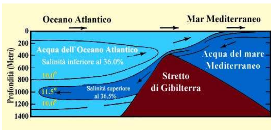
Figura 13: L'acqua del Mediterraneo entra nell'Atlantico tramite lo Stretto di Gibilterra mantenendo inalterate le sue caratteristiche di calore, salinità e minor densità, a causa della barriera che esiste tra i due mari. Le temperature sono in gradi Celsius (C°). ( Marine Geology (Geologia Marina), Kuenen, p. 43, con un piccolo miglioramento.)
