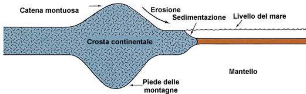
Figura 9: Un'altra illustrazione che mostra come le montagne hanno la forma di pioli, a causa delle loro radici profonde. ( Earth Science (Scienza della Terra), Tarbuck e Lutgens, p. 158.)
